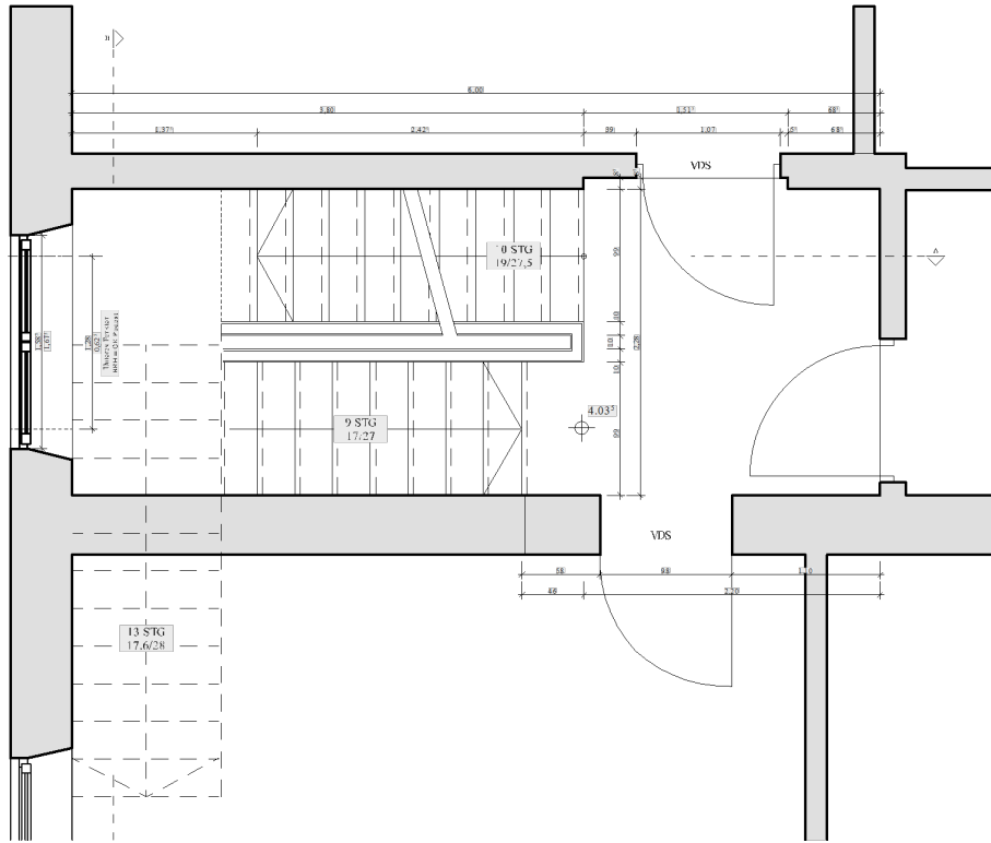
Grundriss DG Treppenhaus Süd
