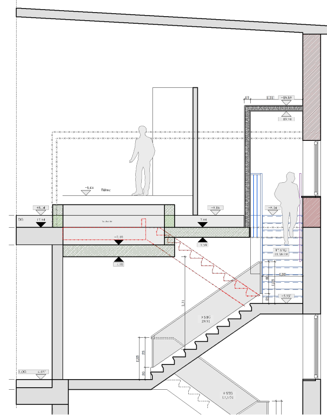
Schnitt 1.OG - DG Treppenhaus Süd
